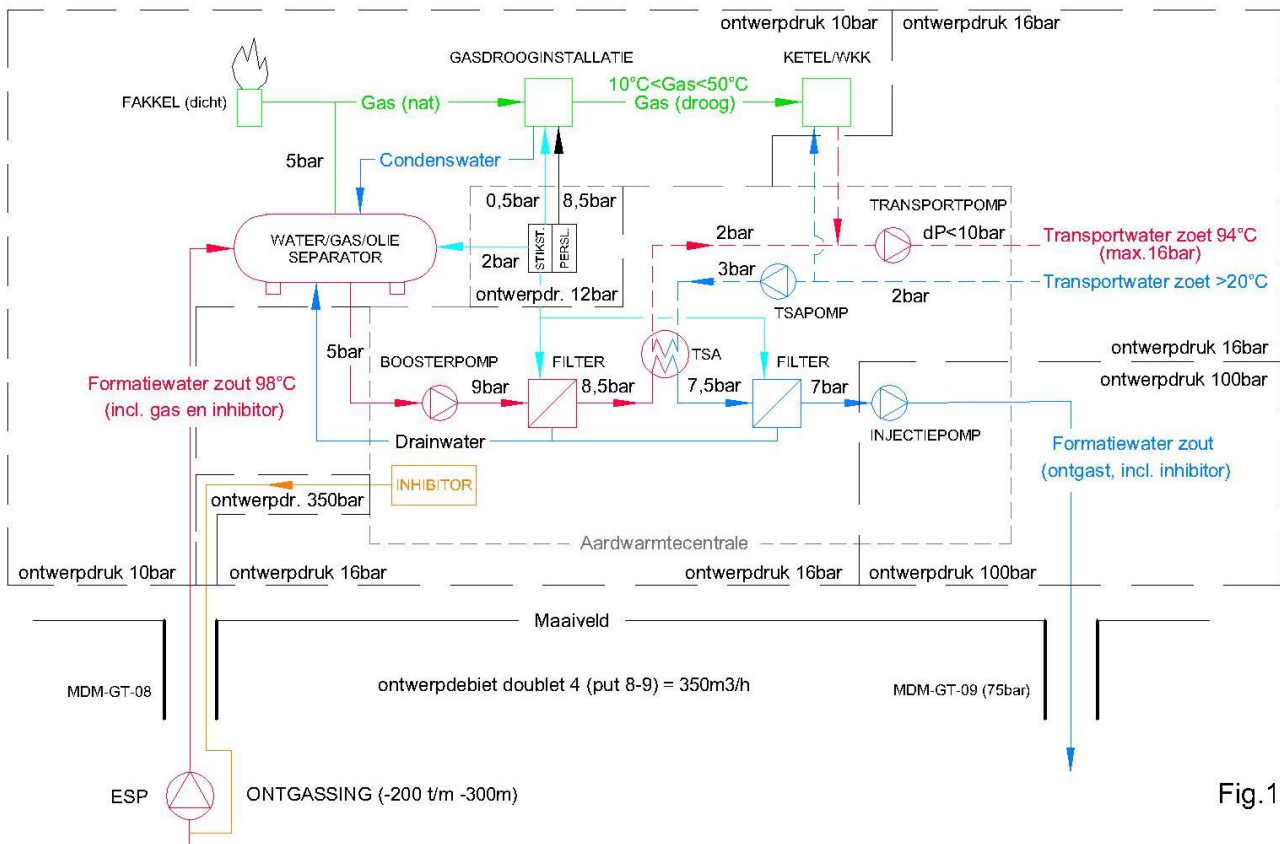
Principeschets Geothermie-installatie ECW-MIT21GEO
